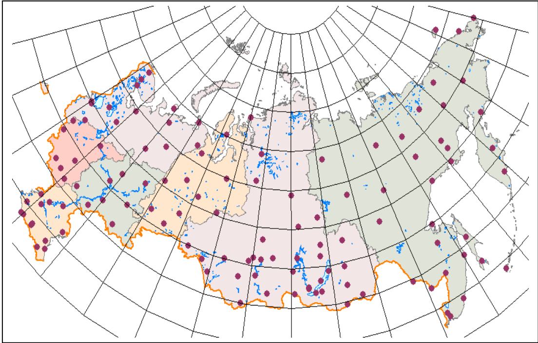
Рис. Станции актинометрической сети, выполняющие наблюдения по полной программе
